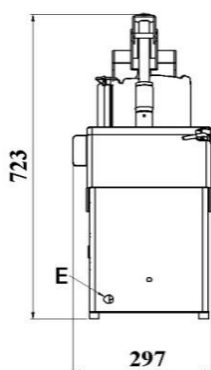
Vista trasera
